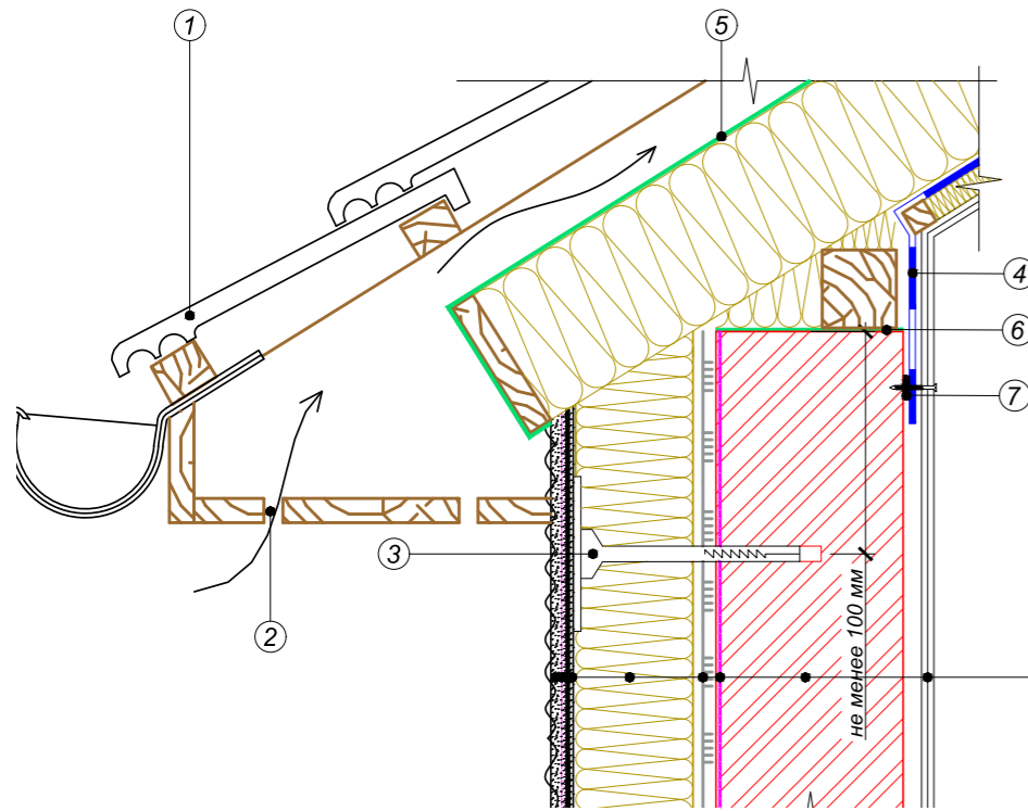
Рисунок 19. Примыкание системы к вентилируемой скатной кровле
