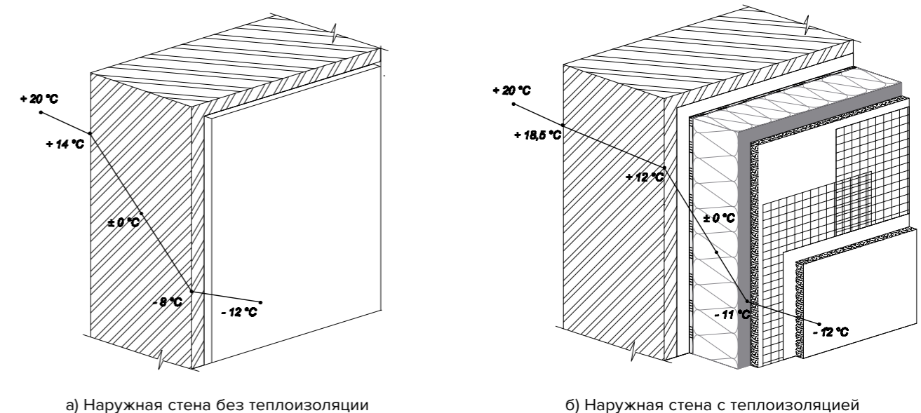
Рисунок 21. Температурная кривая зимой
