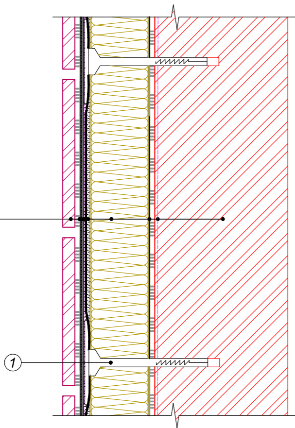
① Тарельчатый фасадный дюбель EJOT H4/H5
