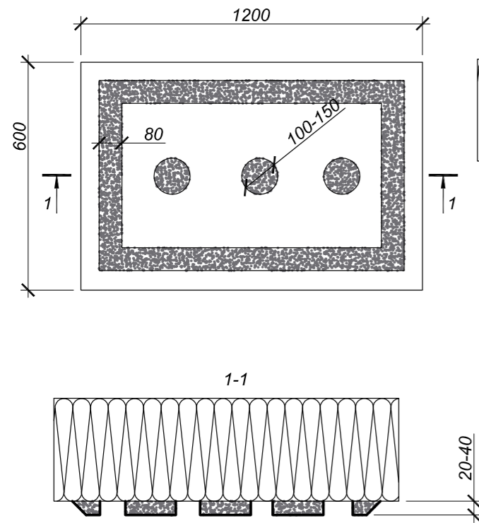
Рисунок 5. Схема точечного нанесения Клеевой смеси для плит из минеральной ваты 110
