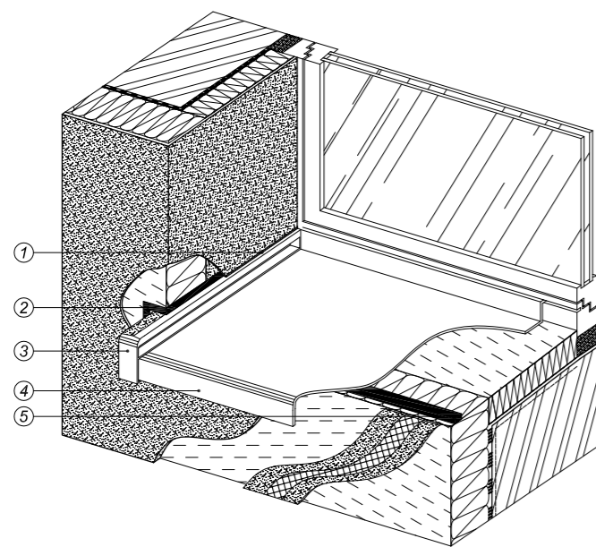
Рисунок 20. Устройство системы в районе оконного отлива
