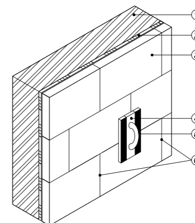
Рисунок 9. Выравнивание поверхности плит
