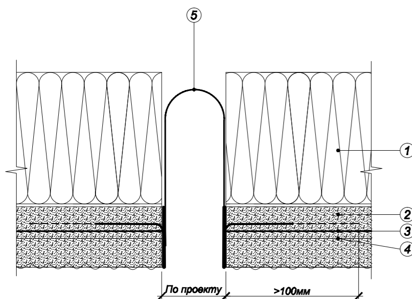
Рисунок 16. Установка компенсатора деформационного шва
