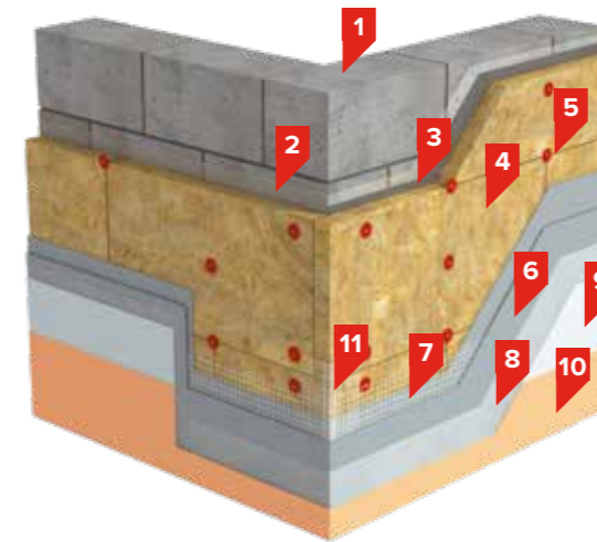
Рисунок 1. Системы с тонким штукатурным слоем
