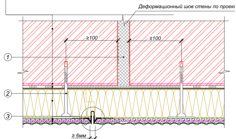
Рисунок 17. Устройство деформационного шва
