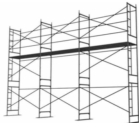
Рисунок 2. Строительные леса
