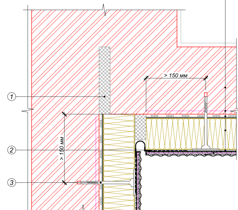
Рисунок 18. Устройство углового деформационного шва
