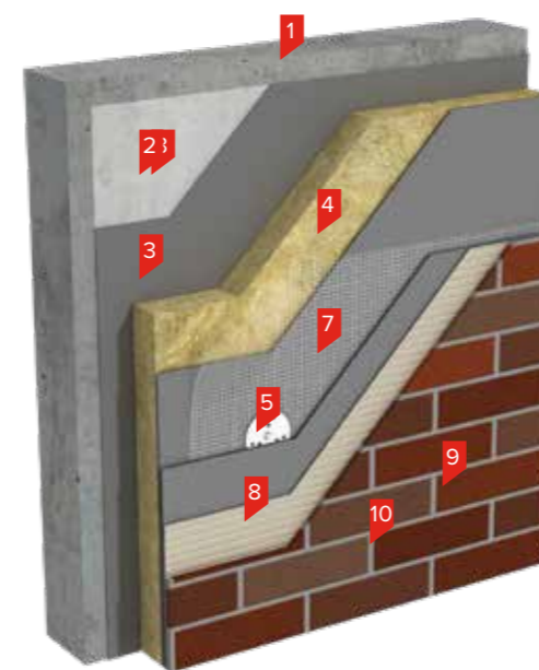
Рисунок 15. Фасадная система с отделкой клинкерной плиткой
