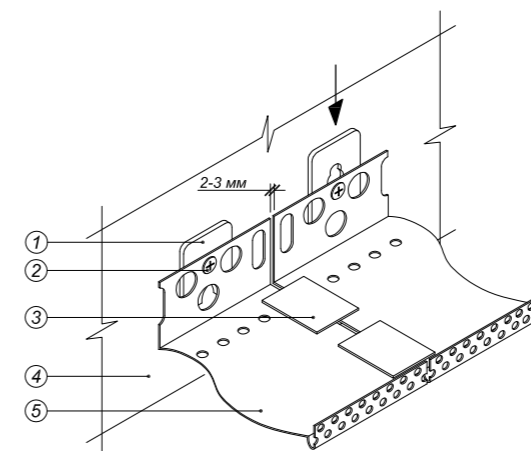
Вариант 1 При монтаже цокольного профиля шириной до 100 мм
